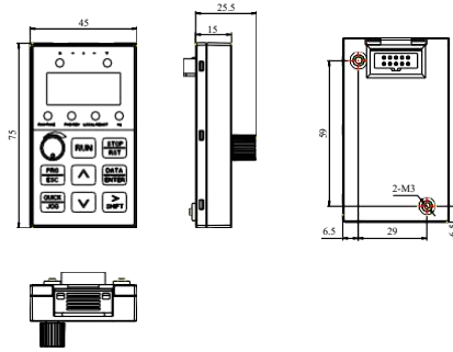
YDL-610系列小键盘外形尺寸
