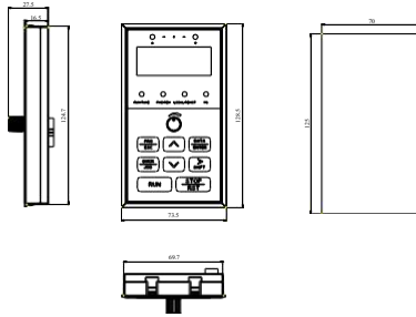
YDL-610系列大键盘外形尺寸
